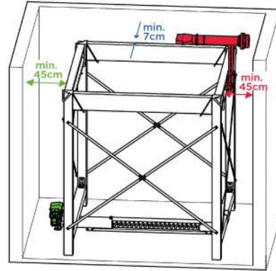
Unidad de llenado, motor de descarga opuesto
